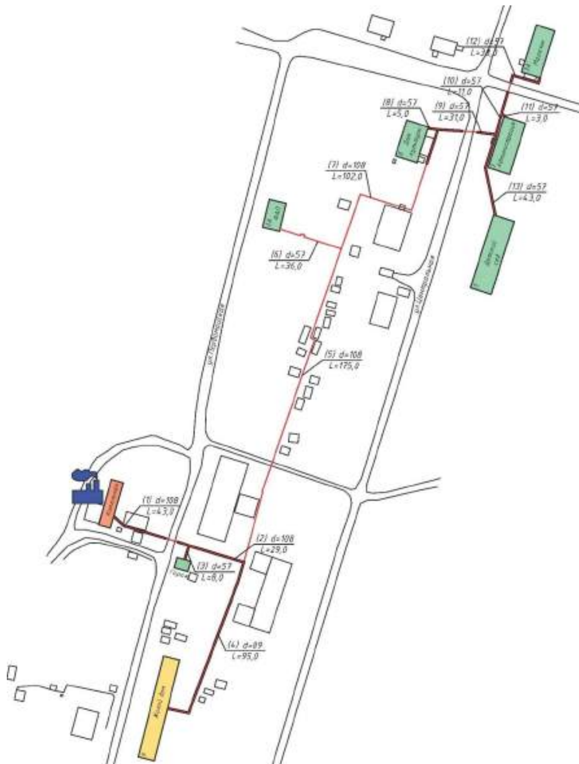
Рисунок 1.3.1. Схема тепловой сети от котельной п.Мирный
