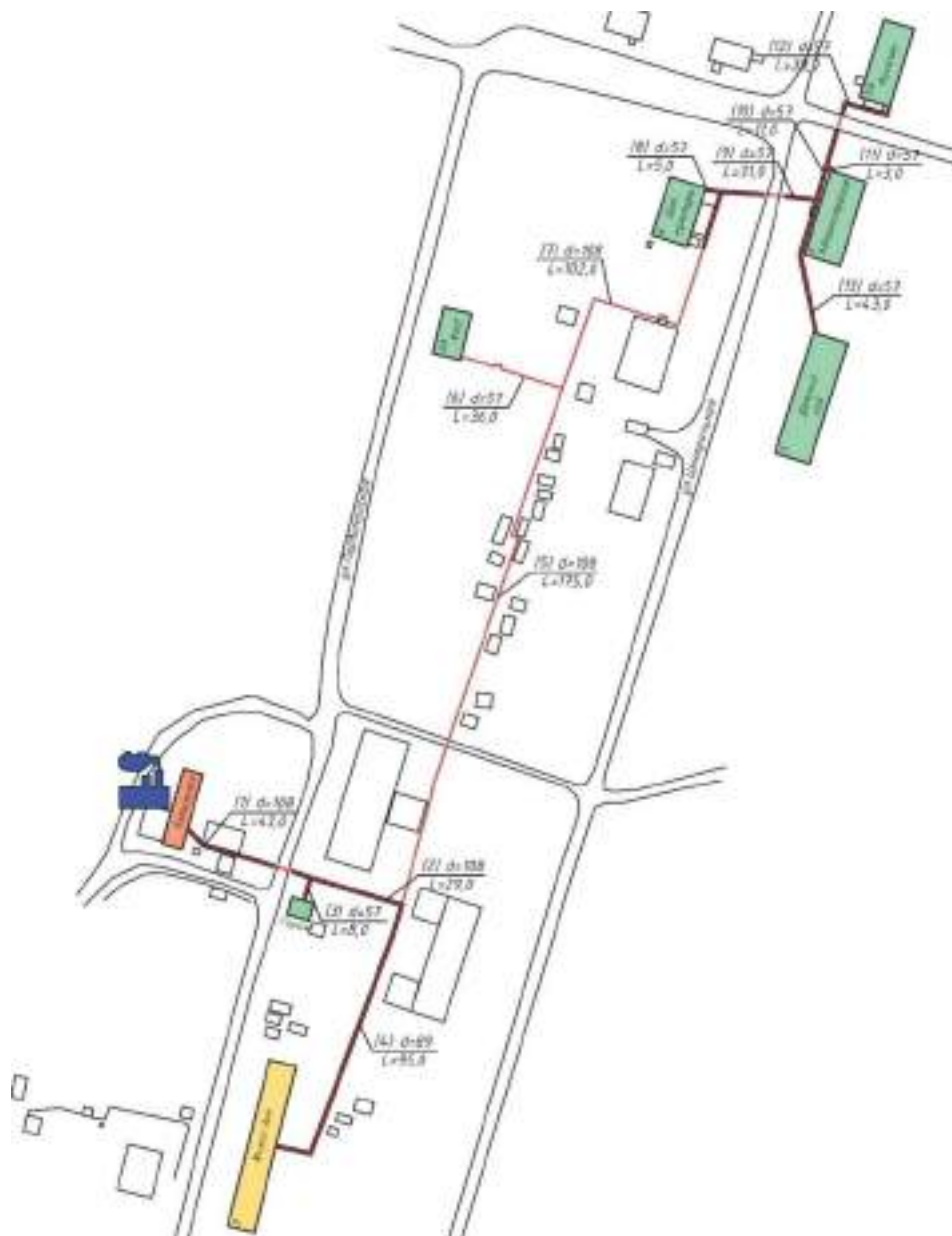
Рисунок 7.1. Схема тепловой сети от котельной п. Мирный
